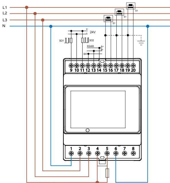
Type 7E.85.8.400.0210
