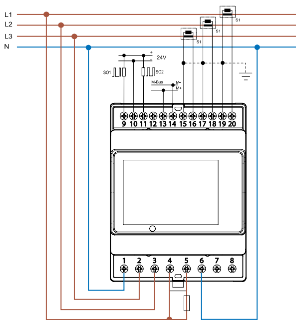
Type 7E.85.8.400.0310
