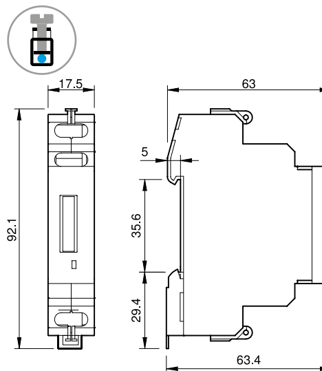
Type 7E.13.8.230.0010 Box clamp
