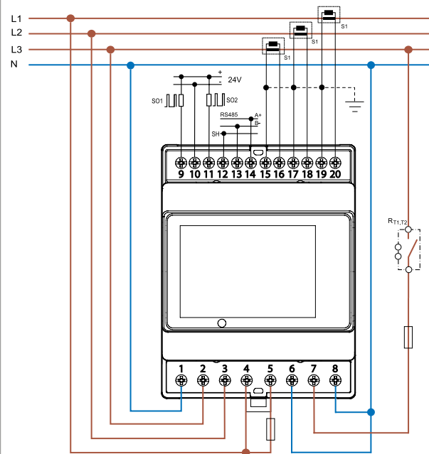
Type 7E.85.8.400.0212
